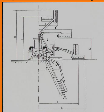
Hydraulische Anfahrssicherung
